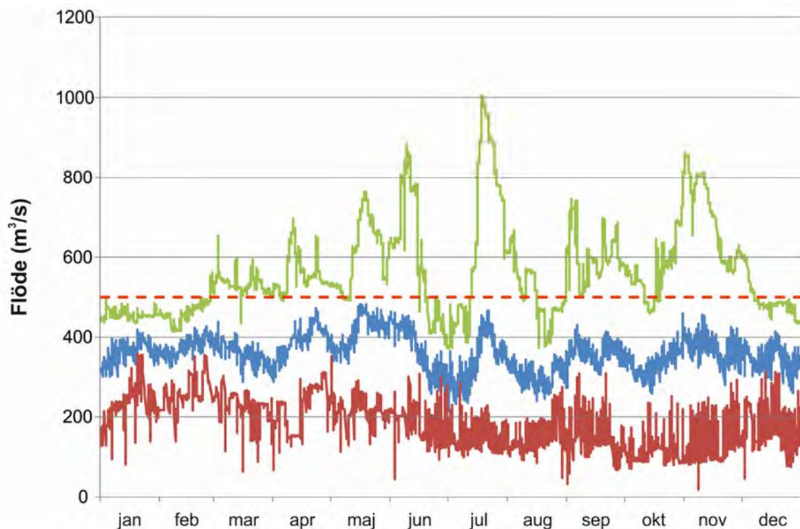
Figur 34. Totalmedelflöde i Söderfors 2011-2016 (blå linje) med 95% konfidensintervall (grön och röd linje). Den röda streckade linjen illustrerar kraftverkets slukförmåga (500 m 3 /s). Flödesdata från Vattenfall (2017).
