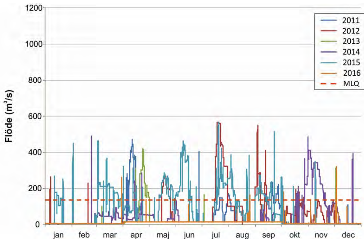
Figur 35. Faktiskt totalt spillflöde vid Söderfors kraftverk 2011-2016. Den röda streckade linjen illustrerar minsta lågvattenföring (MLQ) för Söderfors (135 m 3 /s).
