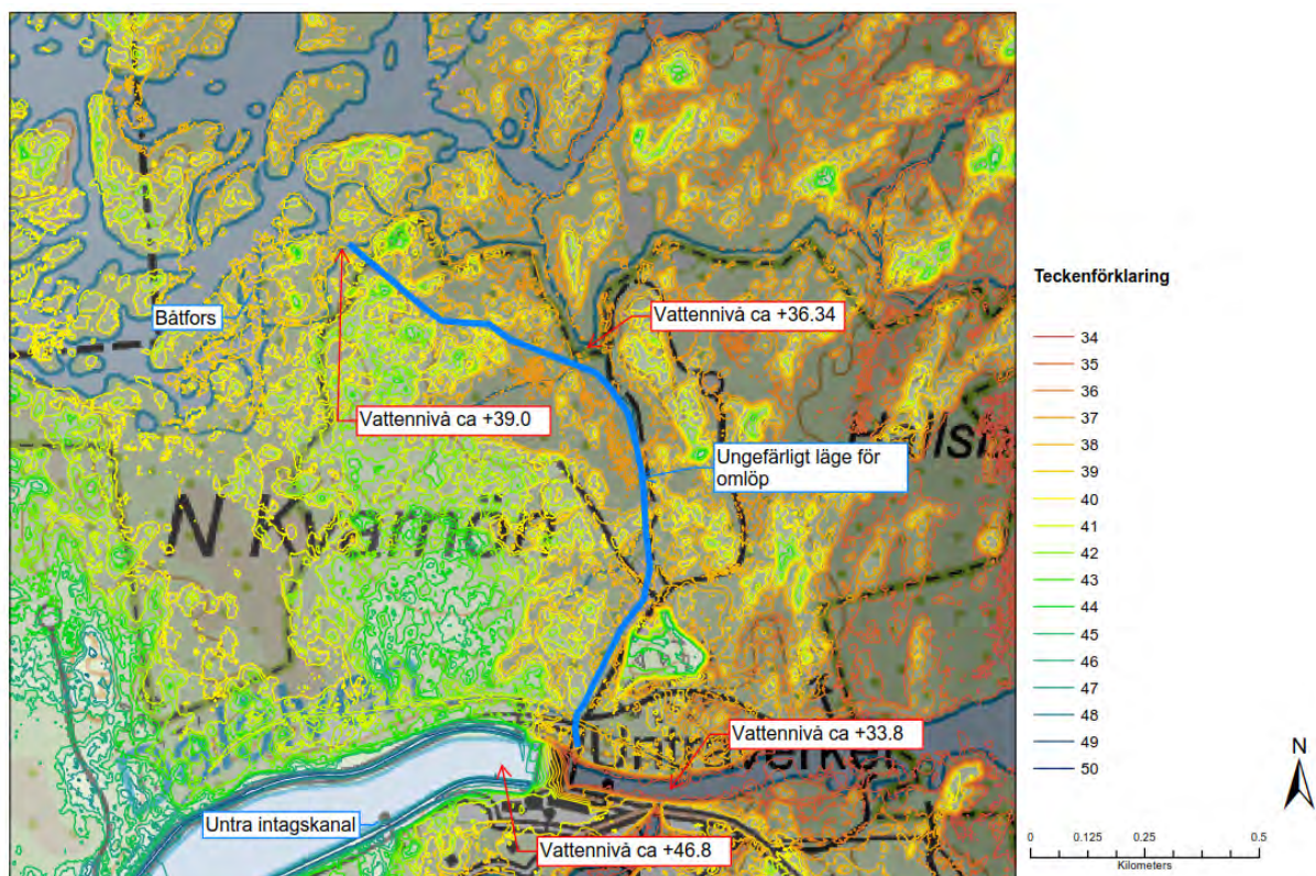
Figur 30. Omlöp mellan Untras utloppskanal och Båtfors. Terrängen är utmarkerad med höjdkurvor.
