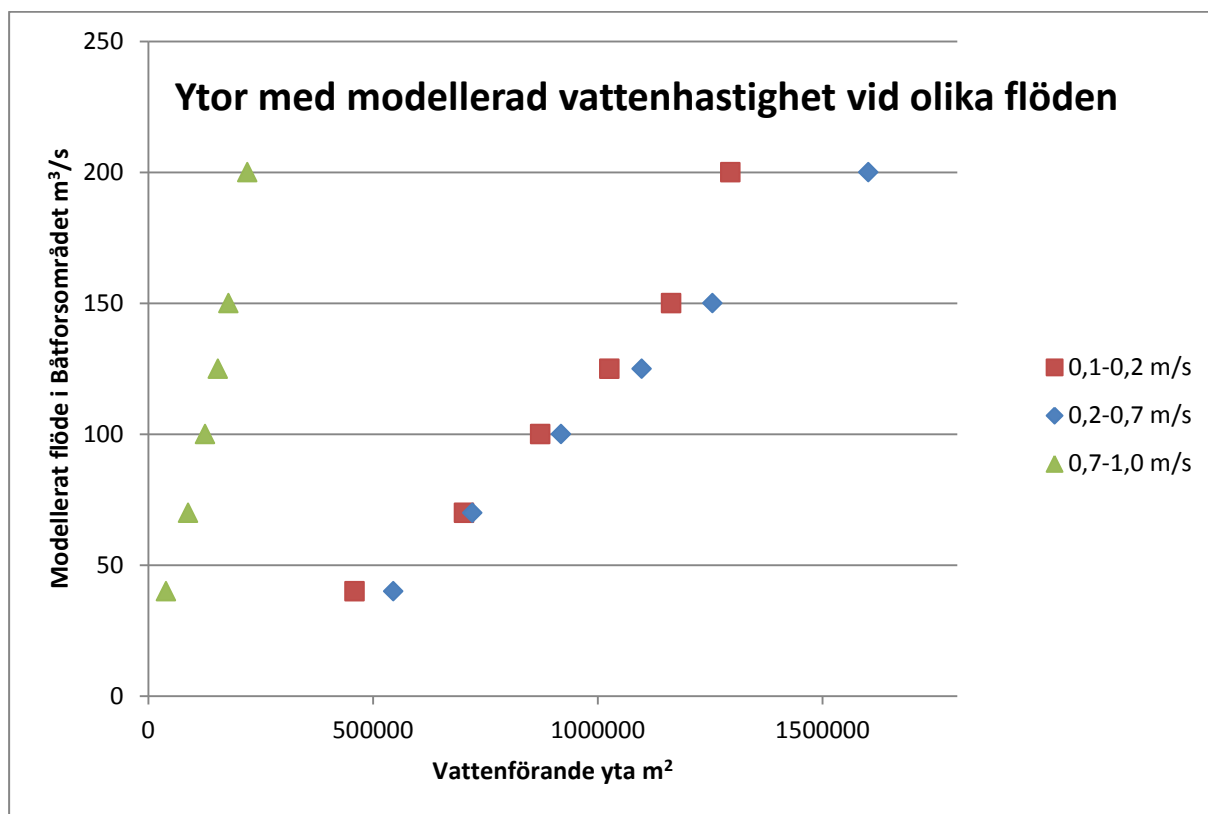
Figur 9. Ytor med beräknad vattenhastighet i Båtforsområdet för de olika beräkningsfallen summerat på olika intervall av vattenhastigheter.
