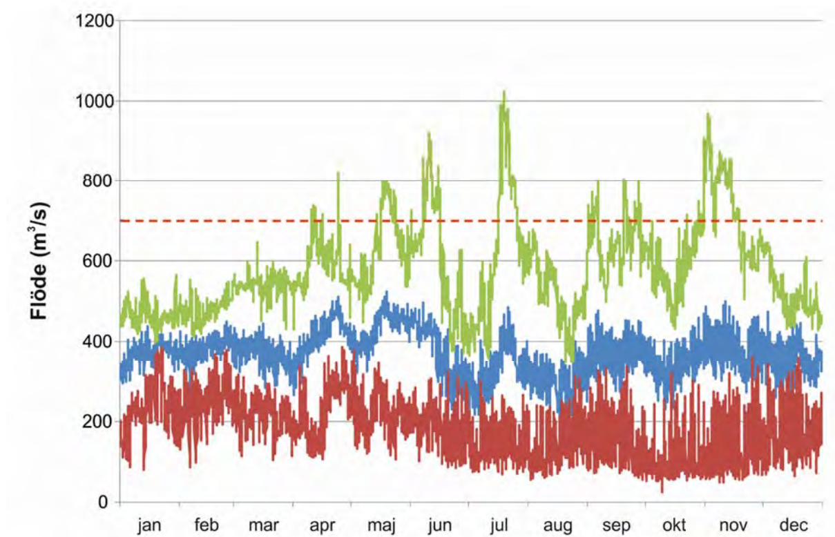
Figur 11. Totalmedelflöde i Älvkarleby 2011-2016 (blå linje) med 95% konfidensintervall (grön och röd linje). Den röda streckade linjen illustrerar kraftverkets slukförmåga. Flödesdata från Vattenfall (2017).
