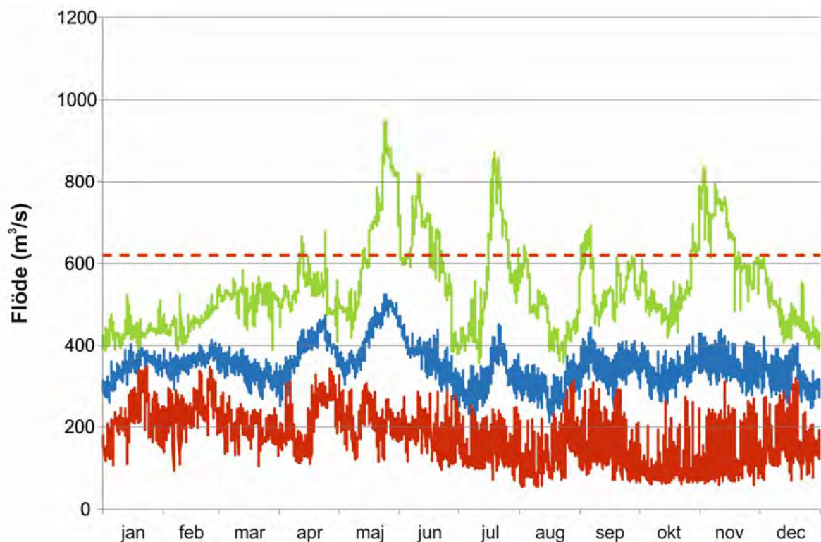
Figur 18. Totalmedelflöde i Lanforsen 2010-2016 (blå linje) med 95% konfidensintervall (grön och röd linje). Den röda streckade linjen illustrerar kraftverkets slukförmåga (620 m³/s). Flödesdata från Fortum (2017).
