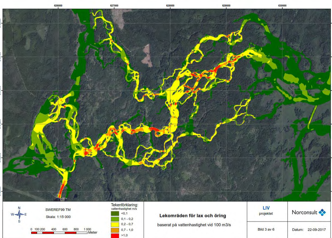
Figur 8. Karta med vattenhastighet för flödet Q 100 .
