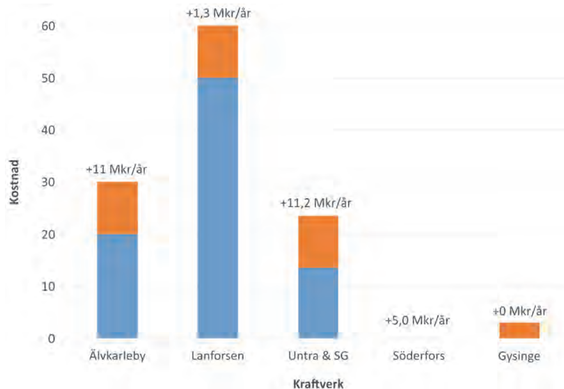
Figur 2. Summering av uppskattade kostnader för rekommenderade åtgärder vid kraftverken i nedre Dalälven. Kostnaderna redovisas som staplar för anläggningskostnader (CAPEX) för uppströms- (blå) och nedströmspassage (orange). Ovanför staplarna anges årliga löpande kostnader (OPEX). Produktion beräknad på ett genomsnittligt elpris om 40 öre/kWh. SG = Storgysingen.
