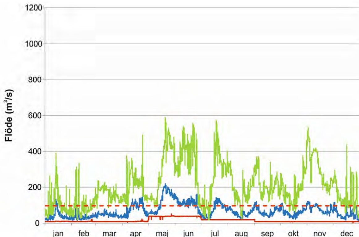
Figur 28. Totalmedelflöde i Båtfors 2010-2016 (blå linje) med 95% konfidensintervall (grön och röd linje). Den röda streckade linjen illustrerar minsta lågvattenföring (MLQ) för Båtfors (108 m³/s) (Hedström-Ringvall et al., 2017). Flödet via Storgysingen är inkluderat. Flödesdata från Fortum (2017).
