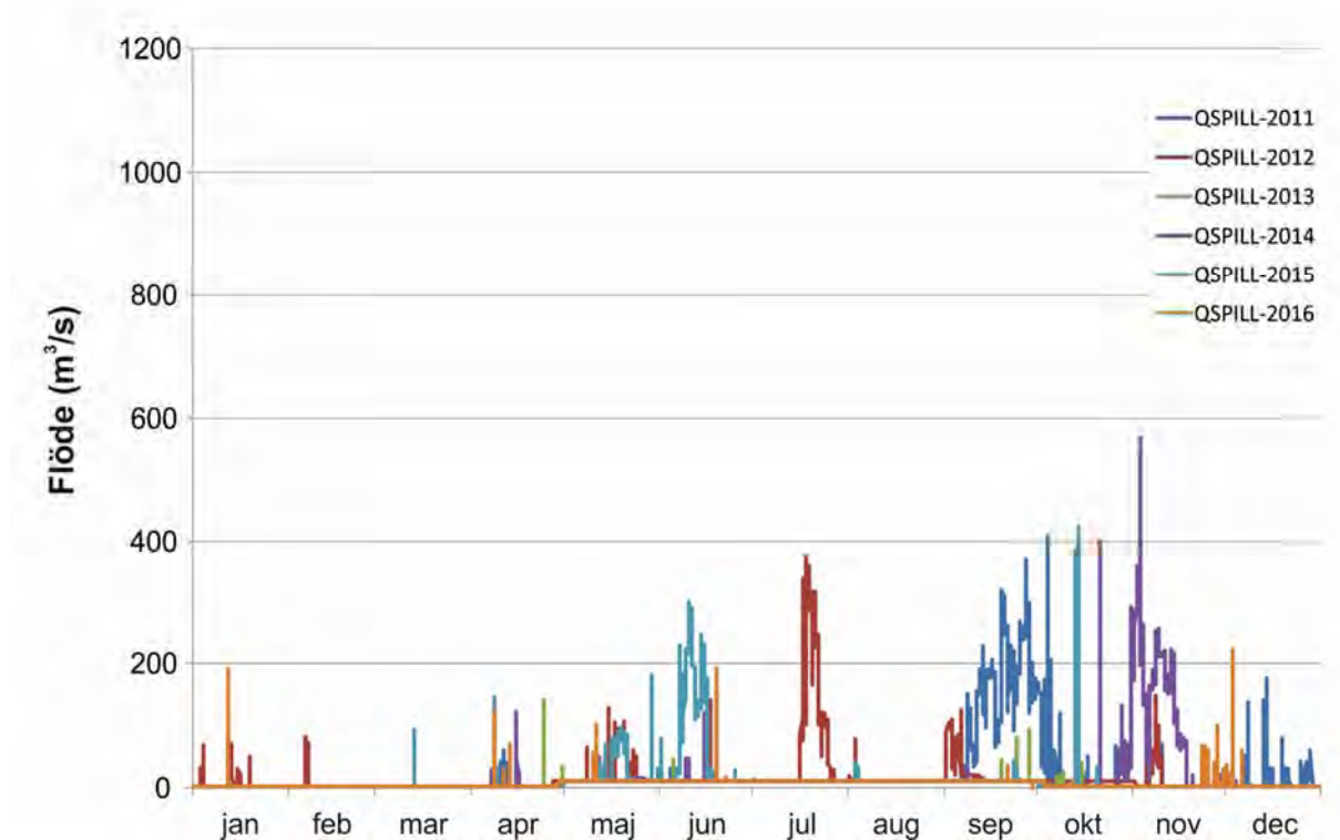
Figur 12. Faktiskt spillflöde vid Älvkarleby kraftverk 2011-2016. Flödesdata från Vattenfall (2017).
