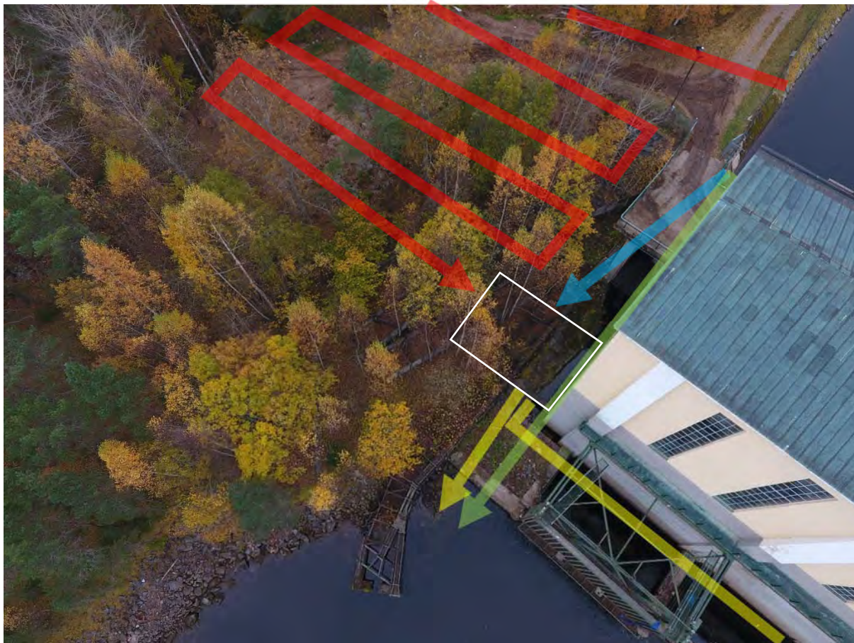
Figur 20. Principskiss över föreslagen dragning av en ny teknisk fiskväg (röd), fiskvägsingångar (gul), placering av dämpningsbassäng (vit), turbinintag minikraftverk (blå) och avledare (grön) vid Lanforsens kraftstation. Norconsult 2017.
