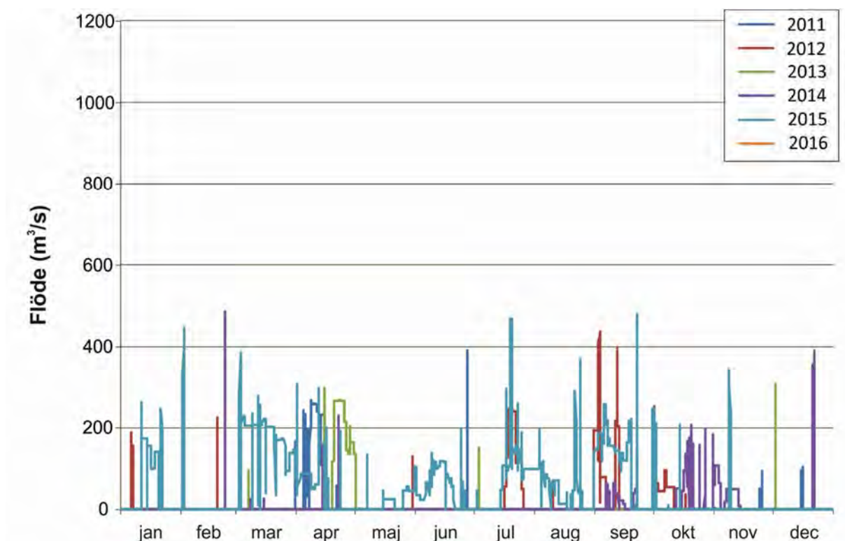
Figur 38. Faktiskt spillflöde i spillluckorna vid Söderfors kraftverk 2011-2016.
