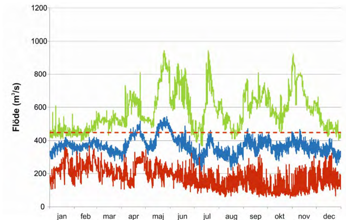
Figur 26. Totalmedelflöde i Untra 2010-2016 (blå linje) med 95% konfidensintervall (grön och röd linje). Den röda streckade linjen illustrerar kraftverkets slukförmåga (450 m³/s). Storgysingen är inte inkluderad eftersom flödet där är att betrakta som spill till Båtfors. Flödesdata från Fortum (2017).
