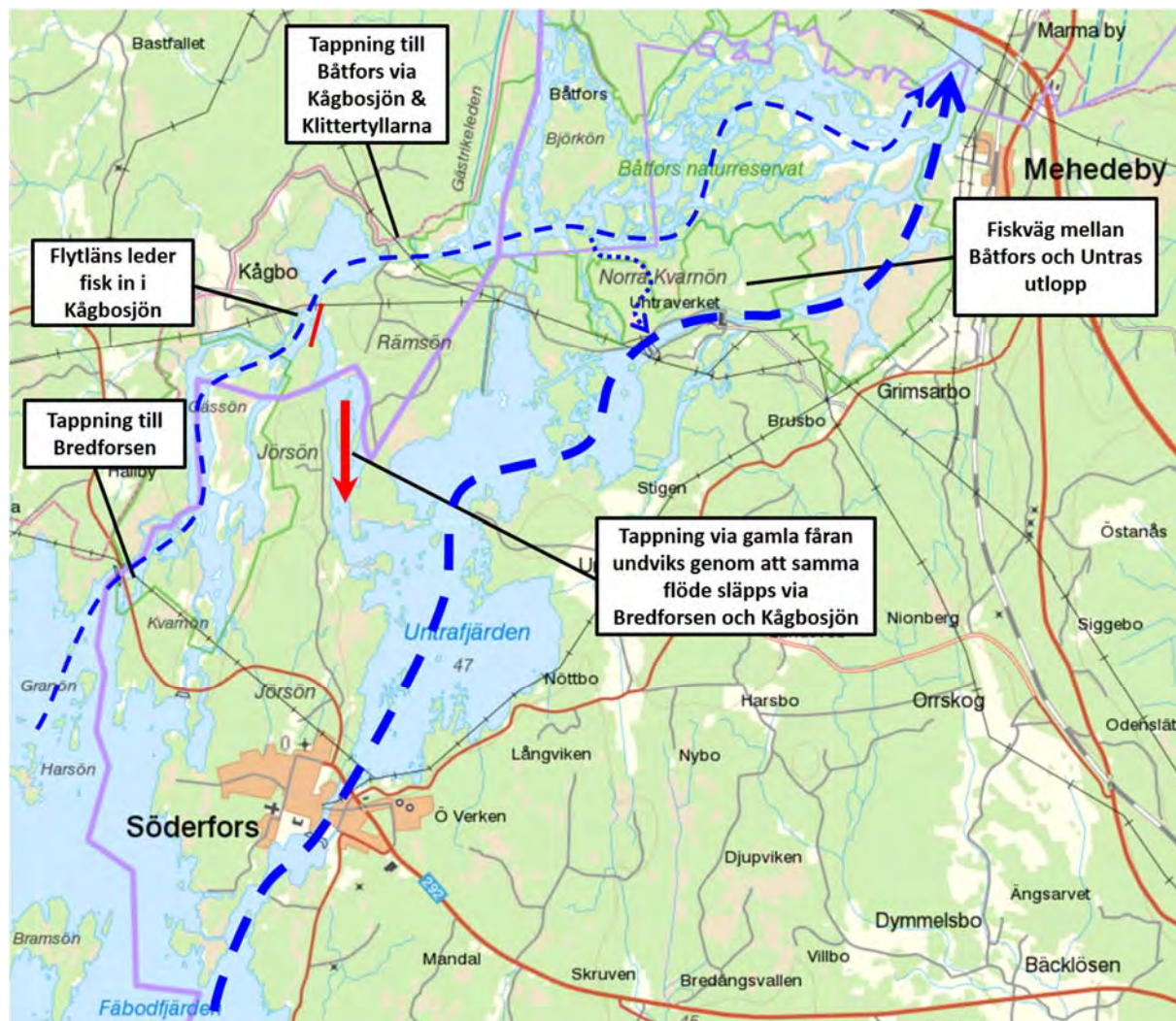
Figur 32. Området i anslutning till Söderfors och Untra kraftverk med översikt av åtgärder och tillhörande strategi för fiskpassage.
