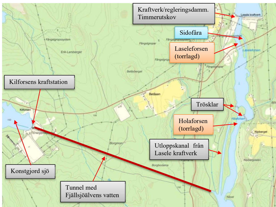
Lasele regleringsdamm och den torrlagda älvfåran.
