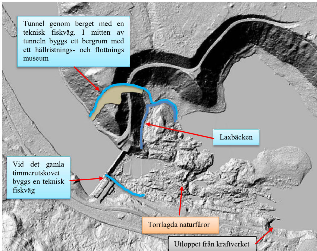
Inlopp till tunneln.
